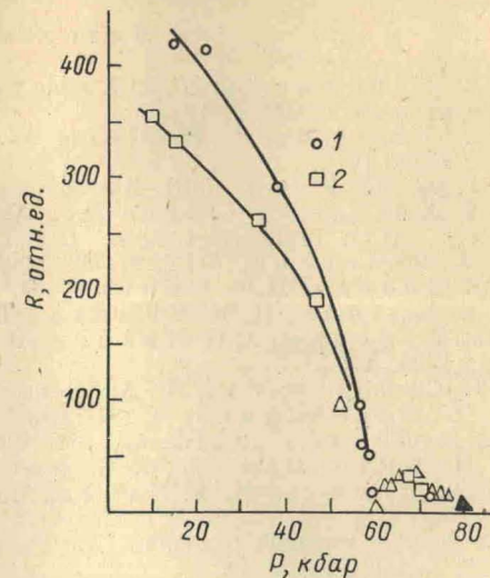
Рис. 2. Постоянная Холла R(P) , взятая при H=70 кЭ, в относительных единицах. 1 — C_3 \parallel H , промежуточная ориентация оси C_3 ; 2 — C_3 \perp H , образец в моноклинной фазе.
