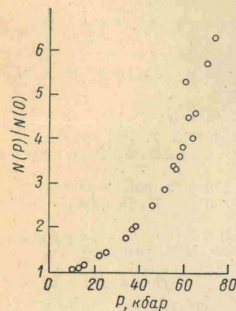
Рис. 1. Концентрация носителей тока в сурьме в зависимости от давления.
